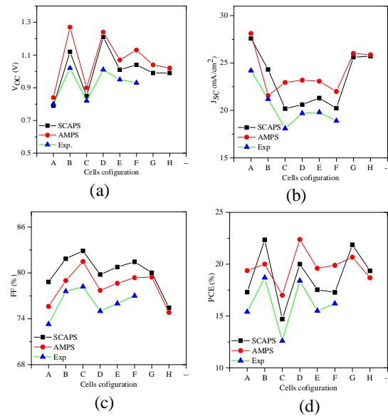
شکل 9. مقایسه اثر سلول‌های خورشیدی پروسکایت با لایه‌های مختلف بر (a): ولتاژ مدار باز (b): چگالی جریان اتصال کوتاه (c): فاکتور پر شدگی (d): بازدهی با استفاده از مقادیر تجربی و نرم افزارهای شبیه‌ساز SCAPS و AMPS.
