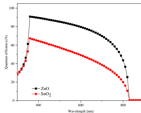
شکل 10. بازده کوآنتومی برحسب طول‌موج نور فرودی برای سلول خورشیدی پروسکایتی با لایه‌های انتقال دهنده الکترون \text{SnO}_2 و \text{ZnO}
