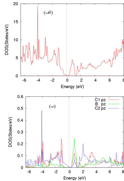
شکل 3. چگالی کل حالت های گرافن با زیرلایه BC_3 و صفحه تک لایه BC_3 . (ب) چگالی حالت های جزئی اوربیتال های Pz اتم های کربن (C2) در گرافن و اتم های کربن (C1) و بورون در صفحه BC_3 .
