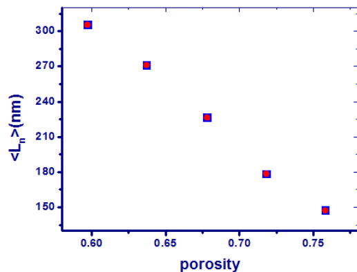
شکل ۴. تغییرات طول پخش الکترون برحسب تخلخل، به ترتیب دایره قرمز مدل حجمی و مربع آبی مدل سطحی تله‌ها را نشان می‌دهند.
